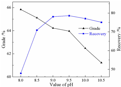
图 4 矿浆 pH 值试验结果 Fig. 4 Test results pf pulp pH value
