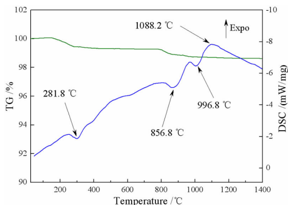
图 4 基础玻璃混合料的热失重 - 差热(TG - DSC)曲线 Fig. 4 TG - DSC curves of basic glass mixture
