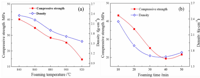
图 5 发泡工艺制度对微晶泡沫玻璃性能的影响(a - 发泡温度,b - 发泡时间)
