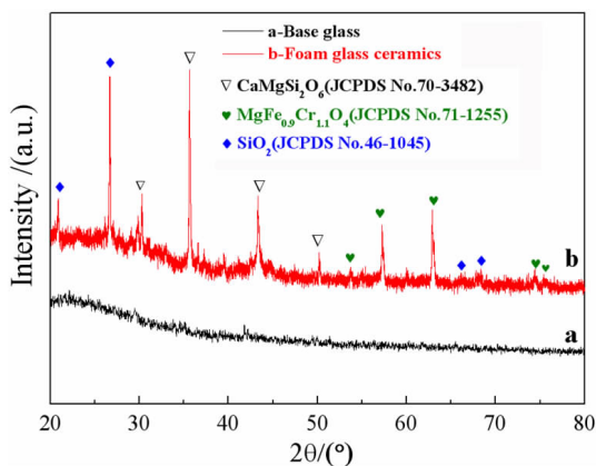
图 3 基础玻璃及微晶泡沫玻璃试样的 XRD 图谱 Fig. 3 XRD patterns of basic glass and foam glass - ceramics
