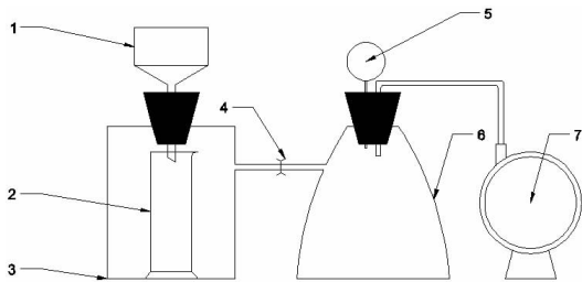
图1 真空过滤试验装置示意图
