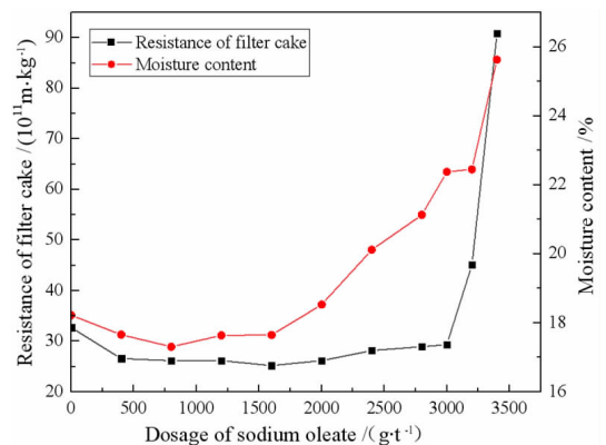
图2 油酸钠用量对赤铁矿精矿滤饼比阻和含水率的影响
