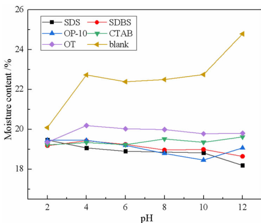
图 8 不同 pH 对赤铁矿精矿含水率的影响 Fig. 8 Effects of pH on the filter cake moisture content of hematite concentrate
