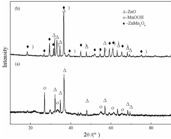
图3 浸出后沉淀与煅烧后沉淀的 X 射线衍射物相分析 Fig. 3 The XRD of the precipitation and calcined precipitation
