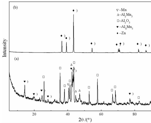
图6 蒸馏获得的锌及还原渣的X射线衍射物相分析 Fig. 6 The XRD of crystalline zinc and reduction slag
