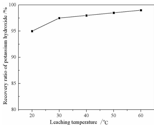
图 2 浸出温度对 KOH 浸出率的影响
