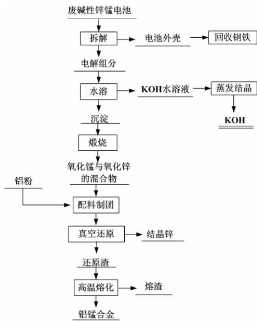
图 1 废旧碱性锌锰电池回收工艺流程
