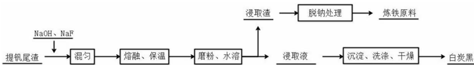
图 3 某提钒尾渣熔盐法制备白炭黑工艺流程
