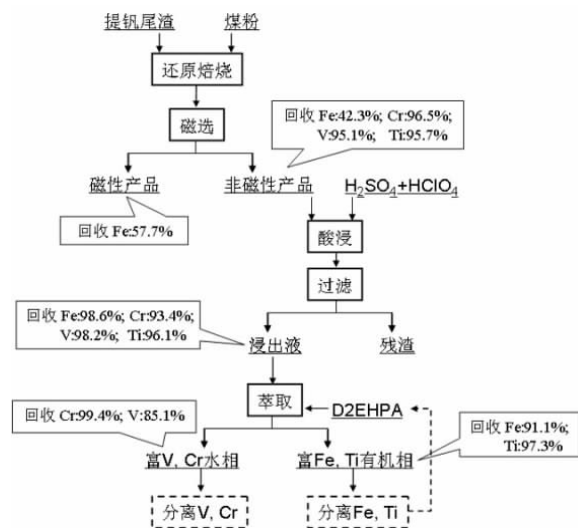
图 2 某提钒尾渣碳热还原法回收有价值元素工艺流程 [32]
