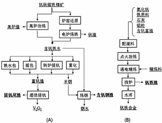
图 1 含钒钢渣(A)和钒铁渣(B)的来源工艺流程
