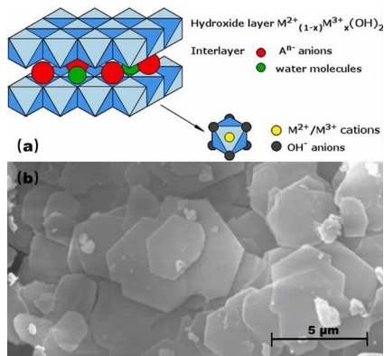
图 1 (a) LDHs 的结构示意图; (b) CaAl - NO 3 LDHs 的 SEM 图 [3,4]
