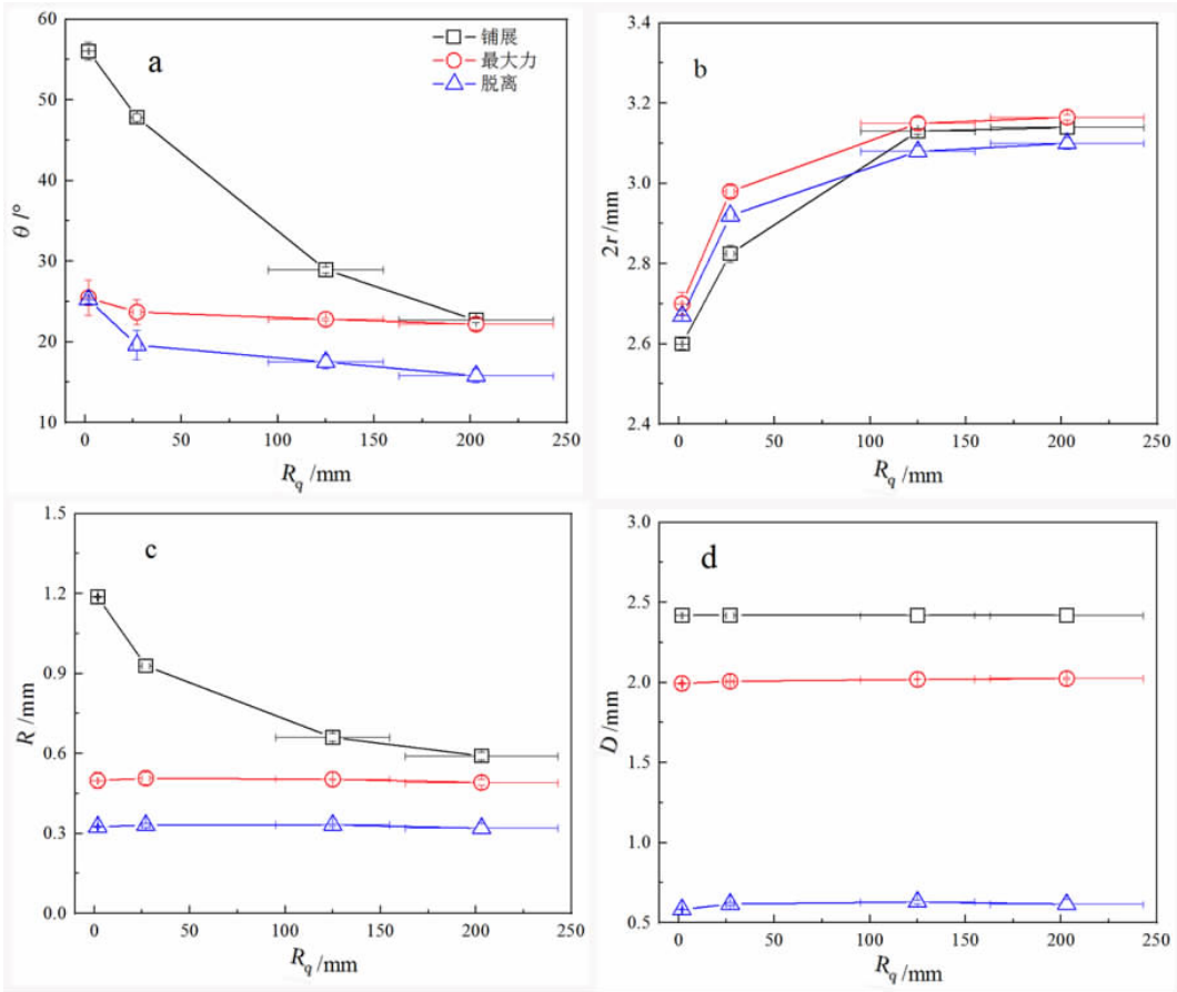
图 5 水滴在天然方解石表面黏附时的形状参数:a,接触角;b,基底直径;c,曲率半径 R ;d,曲率半径 D Fig. 5 The shape parameters of water droplet adhesion on natural calcite surfaces; a, contact angle; b, base diameter; c, curvature radius R ; d, curvature radius D
