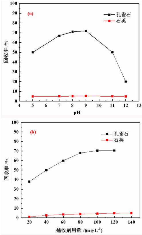
(a) pH 对孔雀石和石英浮选的影响; (b) 邻苯二羟肪酸用量对孔雀石和石英纯矿物捕收性能的影响
