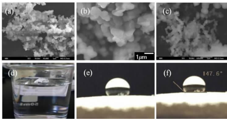
图4 \text{SiO}_2 气凝胶的扫描电镜图(a) (b) (c)和气凝胶的疏水性能(d) (e) (f) [36]
