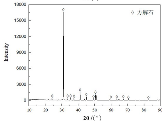
图 2 矿物 X 射线衍射图谱 Fig. 2 The X-ray diffraction pattern of minerals
