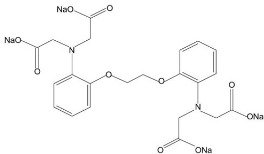
图 1 BAPTA 的结构 Fig. 1 Structure of BAPTA
