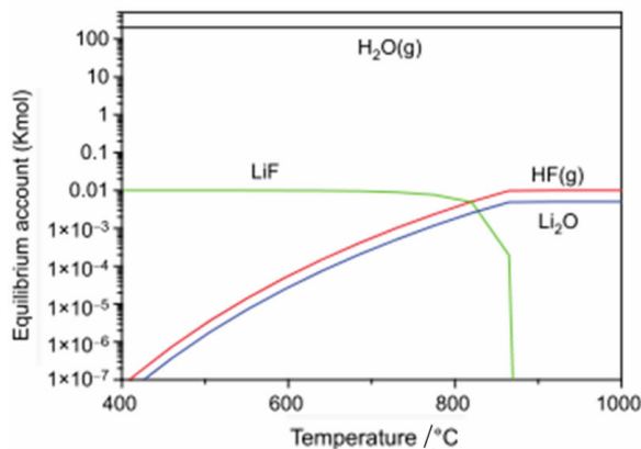
图5 不同温度下 LiF 与水蒸气反应平衡组成 [57]
