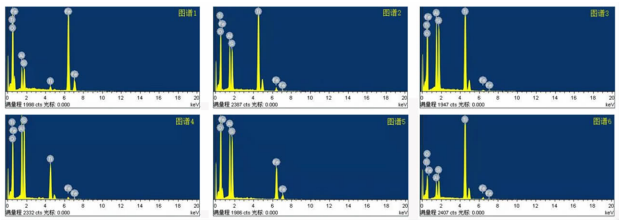
图 4 −0.010 mm 粒级各点 EPMA 能谱分析结果 Fig. 4 EMPA energy spectrum analysis result of −0.010mm classes
