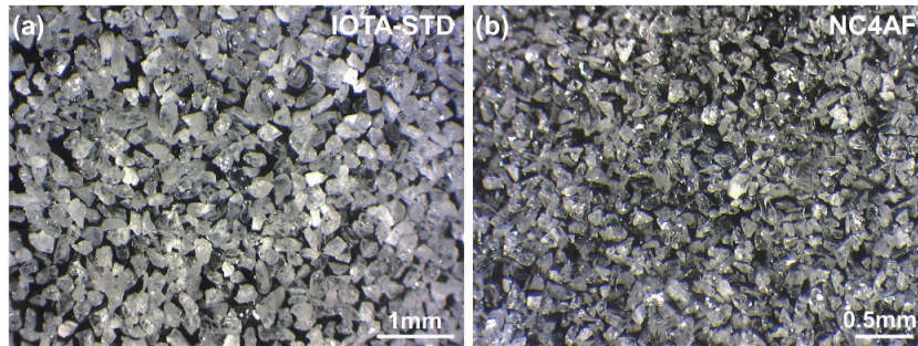
(a)IOTA-STD 为美国 Unimin Corp 生产的 4N8 标准级高纯石英砂, 粒度 40-80 目; (b)NC4AF 为挪威 The Quartz Corp 生产的 4N8 高纯石英砂, 粒度 80-200 目
