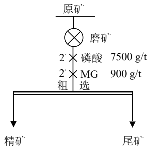
图 1 单一反浮选试验流程(粗选) Fig. 1 Flowsheet of single-reverse roughing flotation tests
