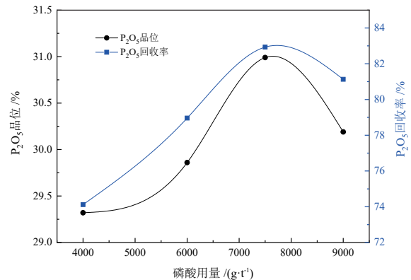
图 3 磷酸用量对精矿品位、回收率的影响 Fig. 3 Results of phosphoric acid dosage tests
