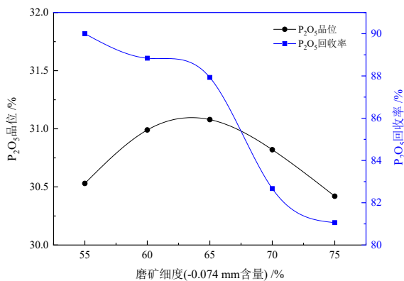
图 2 磨矿细度对精矿品位、回收率的影响 Fig. 2 Results of grinding fineness tests
