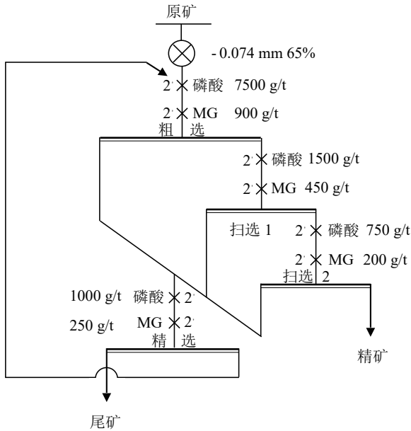
图 5 闭路试验流程 Fig. 5 Flowsheet of closed-circuit test
