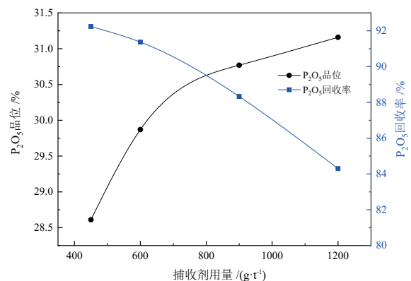
图 4 捕收剂 MG 用量对精矿品位、回收率的影响 Fig. 4 Results of collector MG dosage tests
