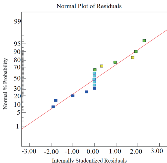
图 8 残差正态分布 Fig. 8 Normal plot of residual error
