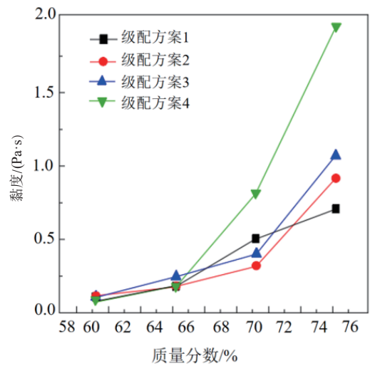
图 2 质量分数对塑性黏度的影响 Fig. 2 Effect of mass fraction on plastic viscosity
