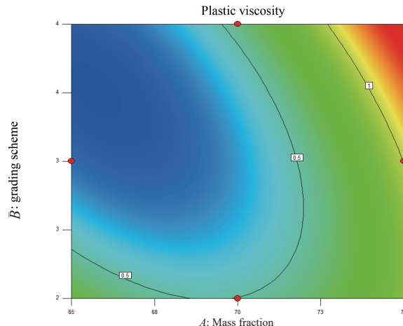
图 9 E=f(A,B) 等高线图 Fig. 9 E=f(A,B) contour map
