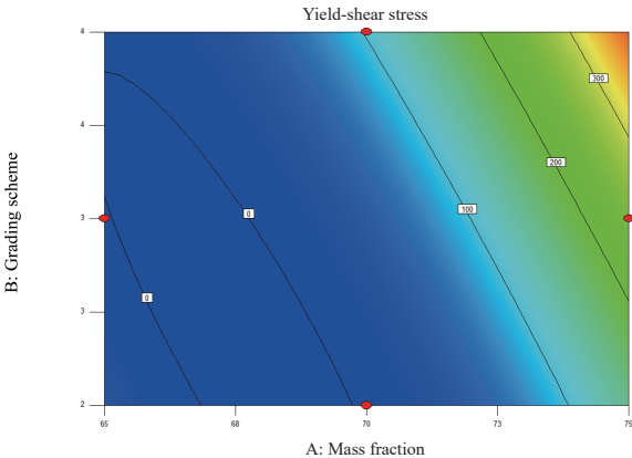
图 6 D=f(A,B) 等高线图 Fig. 6 D=f(A,B) contour map
