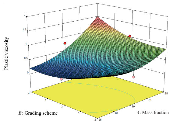
图 10 E=f(A,B) 响应面图 Fig. 10 E=f(A,B) response surface diagram
