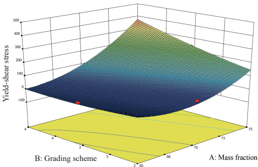
图 7 D=f(A,B) 响应面图 Fig. 7 D=f(A,B) response surface diagram
