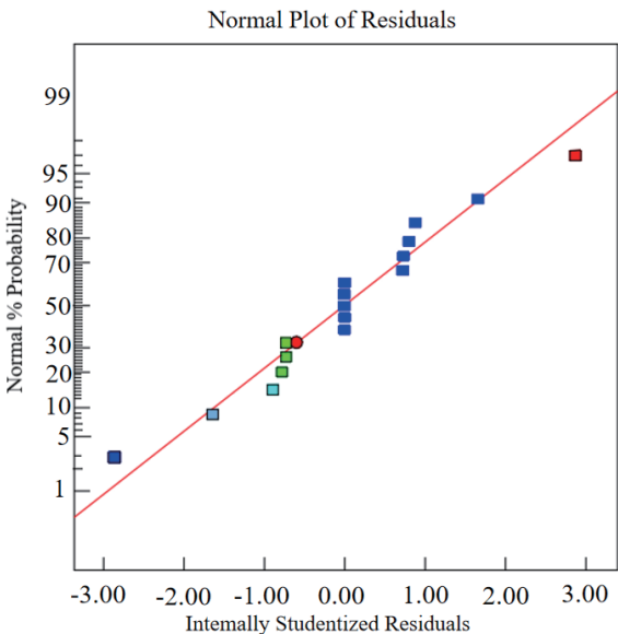
图 5 残差正态分布 Fig. 5 Normal plot of residual error
