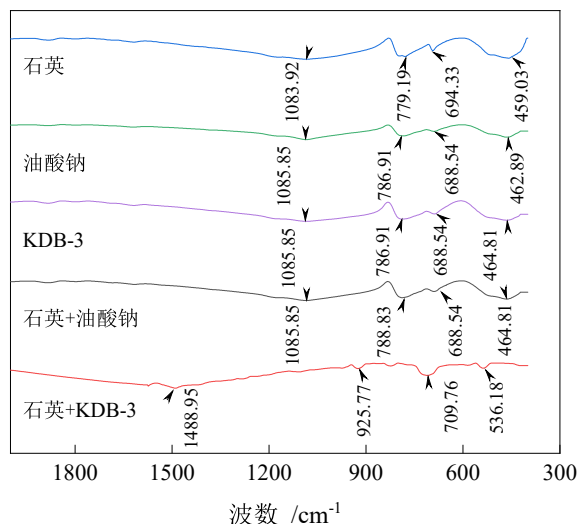
图 7 药剂与石英作用后的红外光谱图
