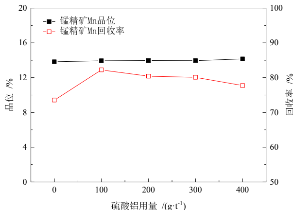
图 4 硫酸铝用量实验结果
