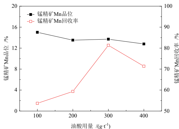
图 5 油酸用量实验结果
