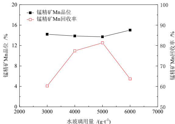
图 3 水玻璃用量实验结果
